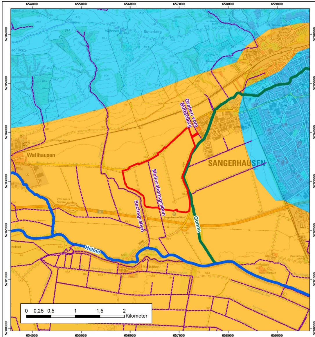
Abbildung 31 Abgrenzung der Grund- und Oberflächenwasserkörper in der Umgebung des Geltungsbereichs
