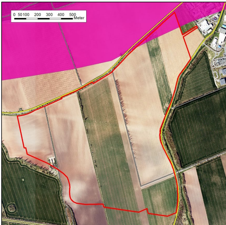
Abbildung 6 Bewertung der Archivfunktion (nach BFBV-LAU)
