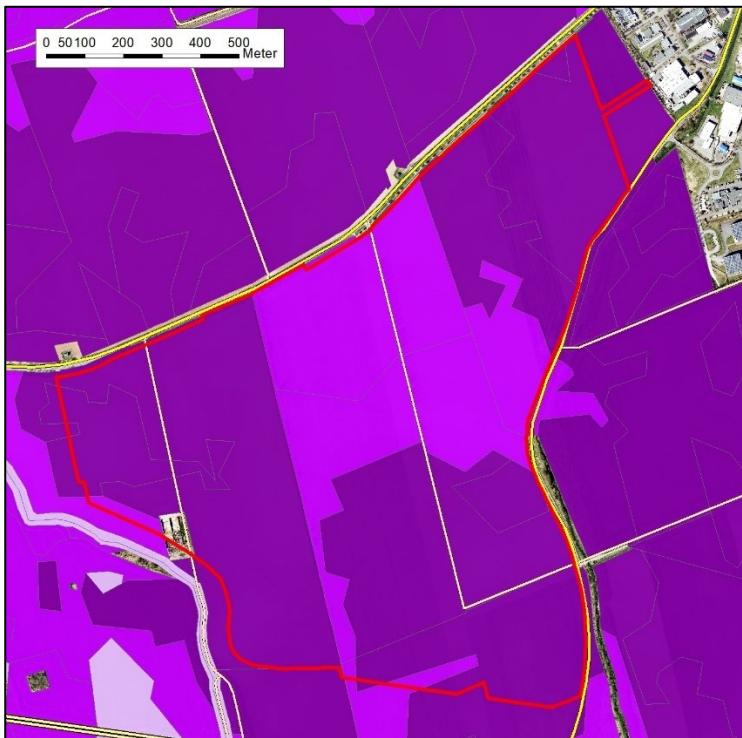
Abbildung 5 Bewertung der Funktionen im Wasserhaushalt (nach BFBV-LAU)
